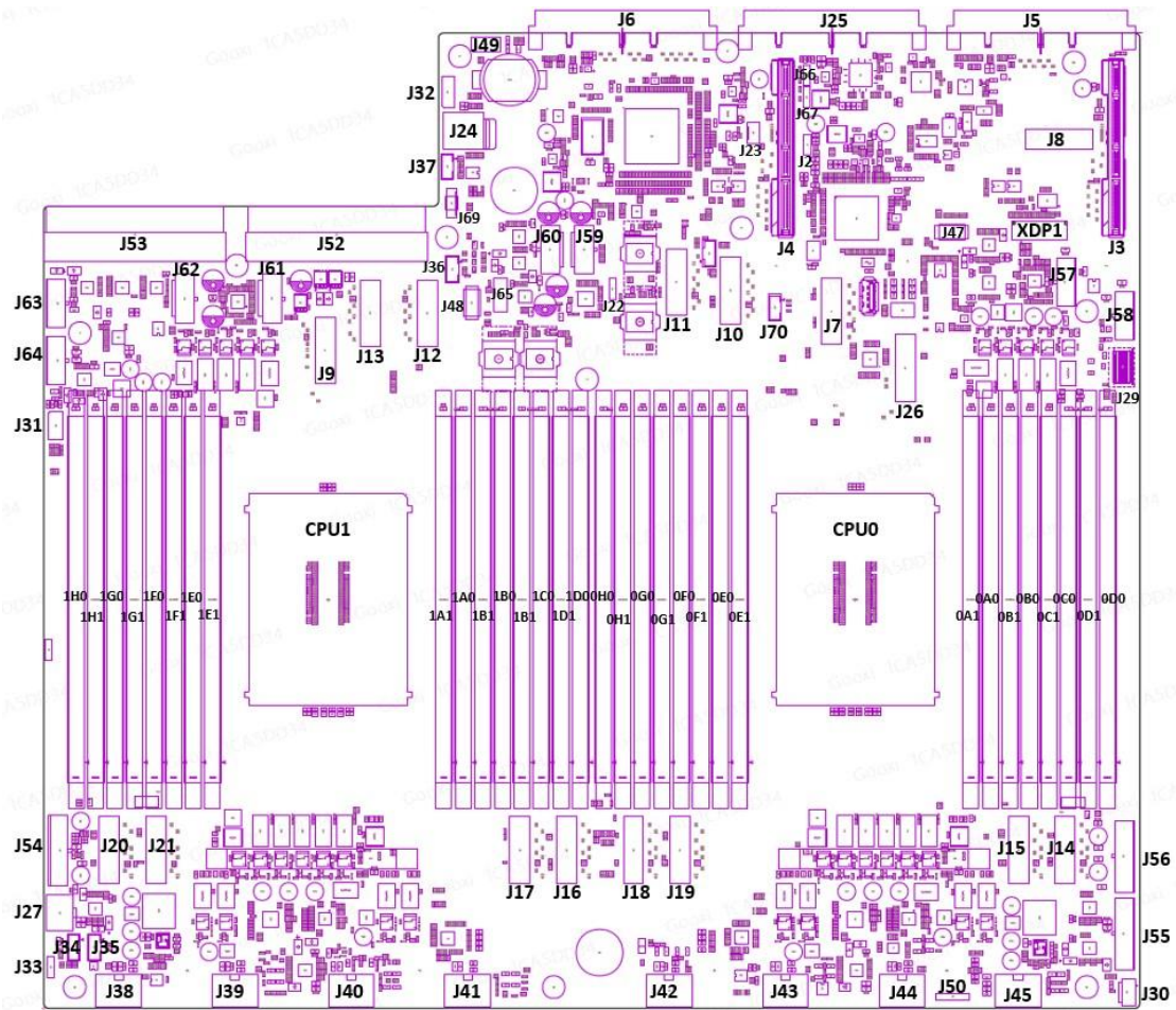
主板图 2-20
