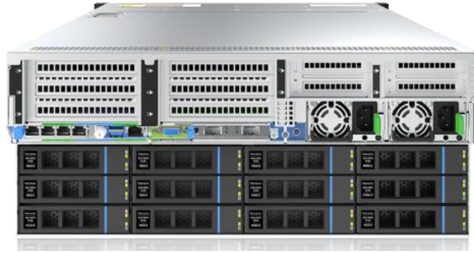
机型后视图
